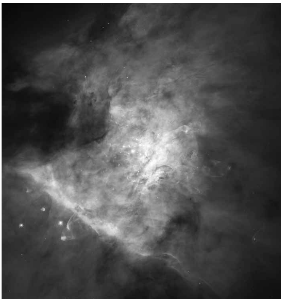
5. Lebensphase: bereits erkaltete Staubmassen, auf welche heisse Filamente stossen und mit welchen sie in Äonen-langer Auseinandersetzung schliesslich wieder neue Formen verdichteter Materie bilden (OrionNebel-VIS) [Bild: NASA]
