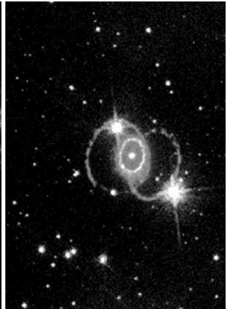
4. Lebensphase: ein schwerer Stern, der sich mit seiner Supernova-Explosion in einem letzten Feuerwerk von der Bühne der Hellen verabschiedet und dabei sein ganzes Vermögen in Form von heissem Gas aus neugeschmiedeten Metallen an die Umgebung zurückgibt (SN 1987A) [Bild: NASA]
