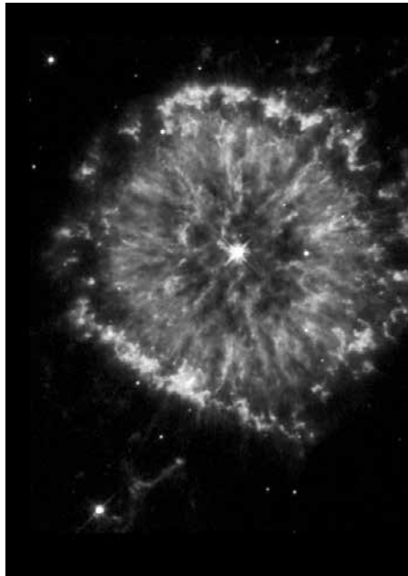
3. Lebensphase: das sanfte Abschütteln der äusseren Hüllen zum «Planetarischen Nebel» im angehenden Alter (NGC 6751) [Bild: NASA]
